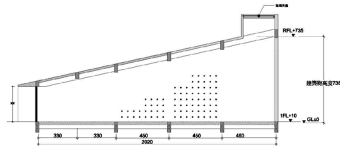
02 AP-02 B 向剖面圖
