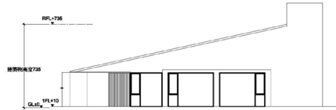
04 AP-02 側向立面圖一
