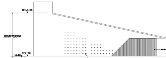
06 AP-02 側向立面圖一
