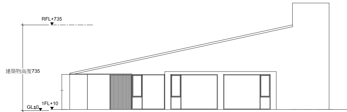
04 AP-02 側向立面圖一
