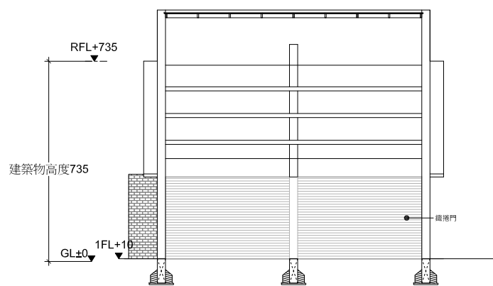
01 AP-02 A向剖面圖
