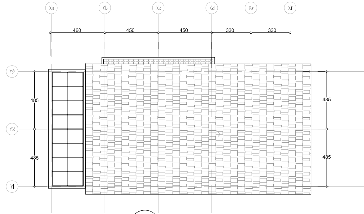
03 AP-01 屋頂平面圖
