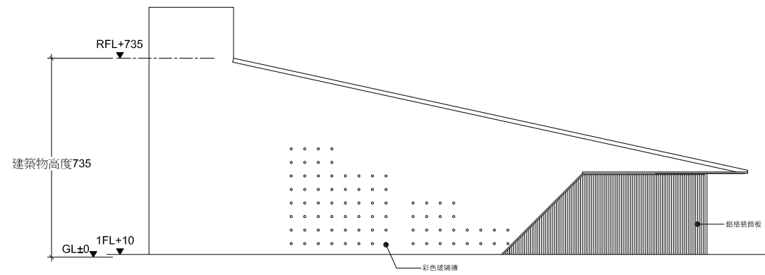
06 AP-02 側向立面圖一
