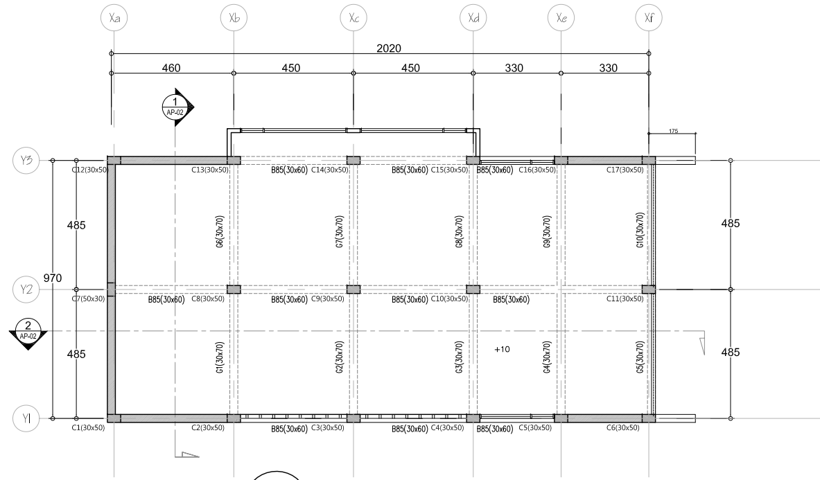
02 AP-01 一層平面圖
