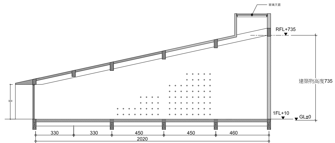
02 AP-02 B向剖面圖
